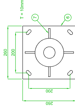
Base plate / Chân đế M16 x 500
